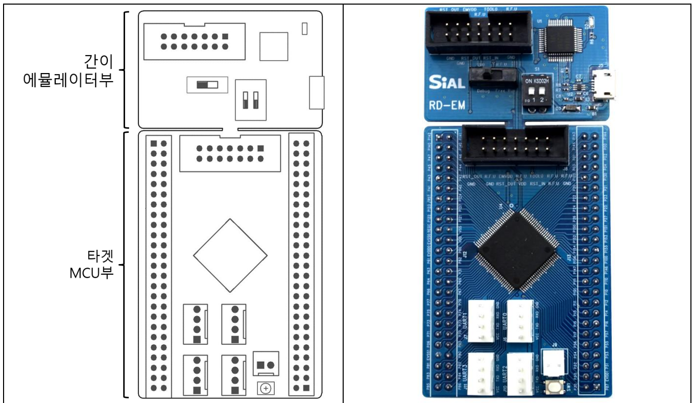
그림 1-1 100P 모델의 외관
