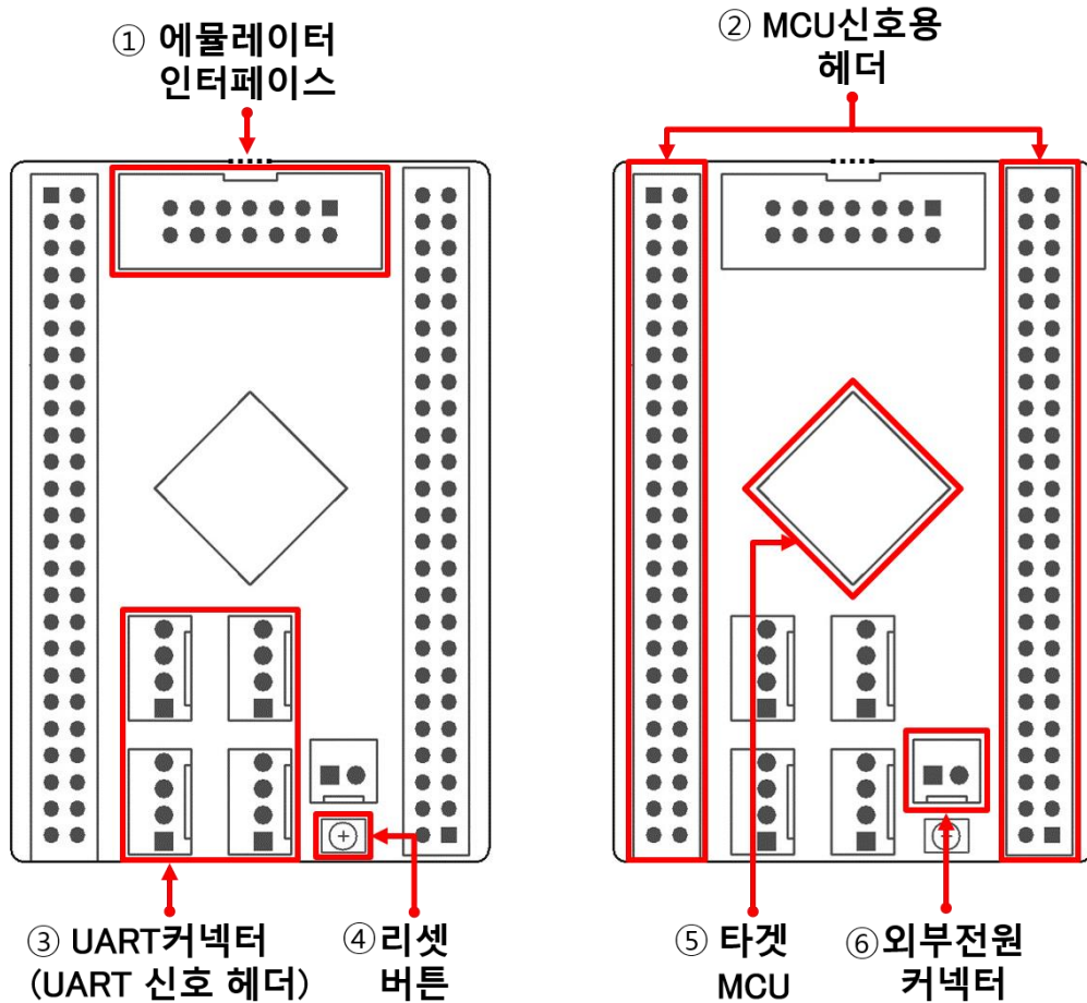
그림 3-1 타겟 MCU 부의 주된 부품배치
