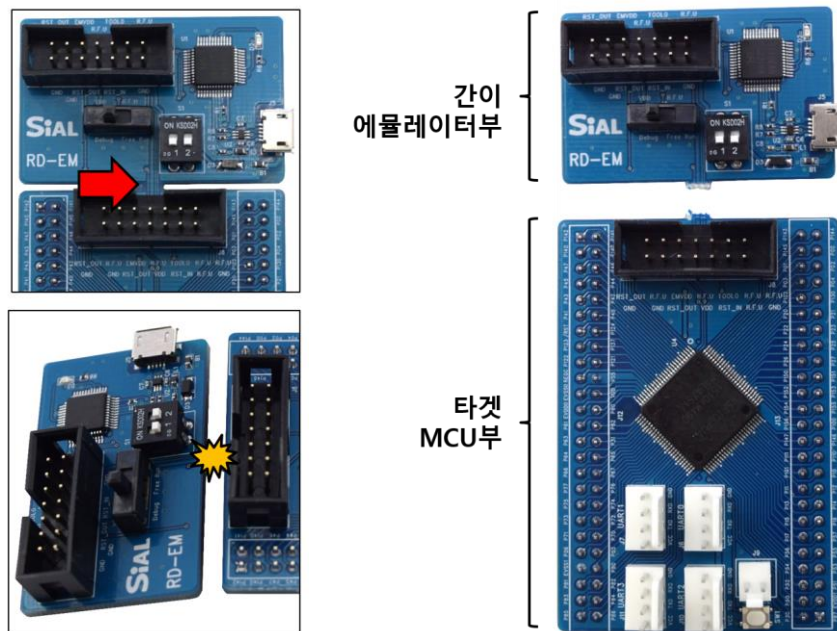
그림 4-1 보드 분리 시 사진
