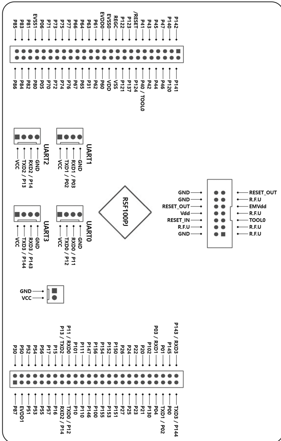
그림 7-1 100P 모델의 커넥터 및 신호 배치
